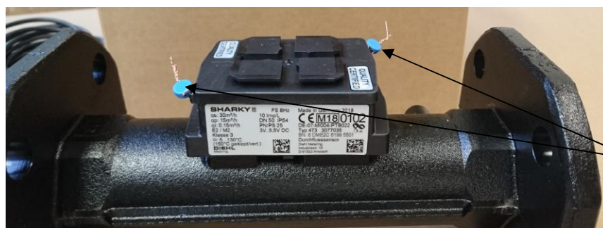
Рисунок 2 – Схема пломбировки от несанкционированного доступа
