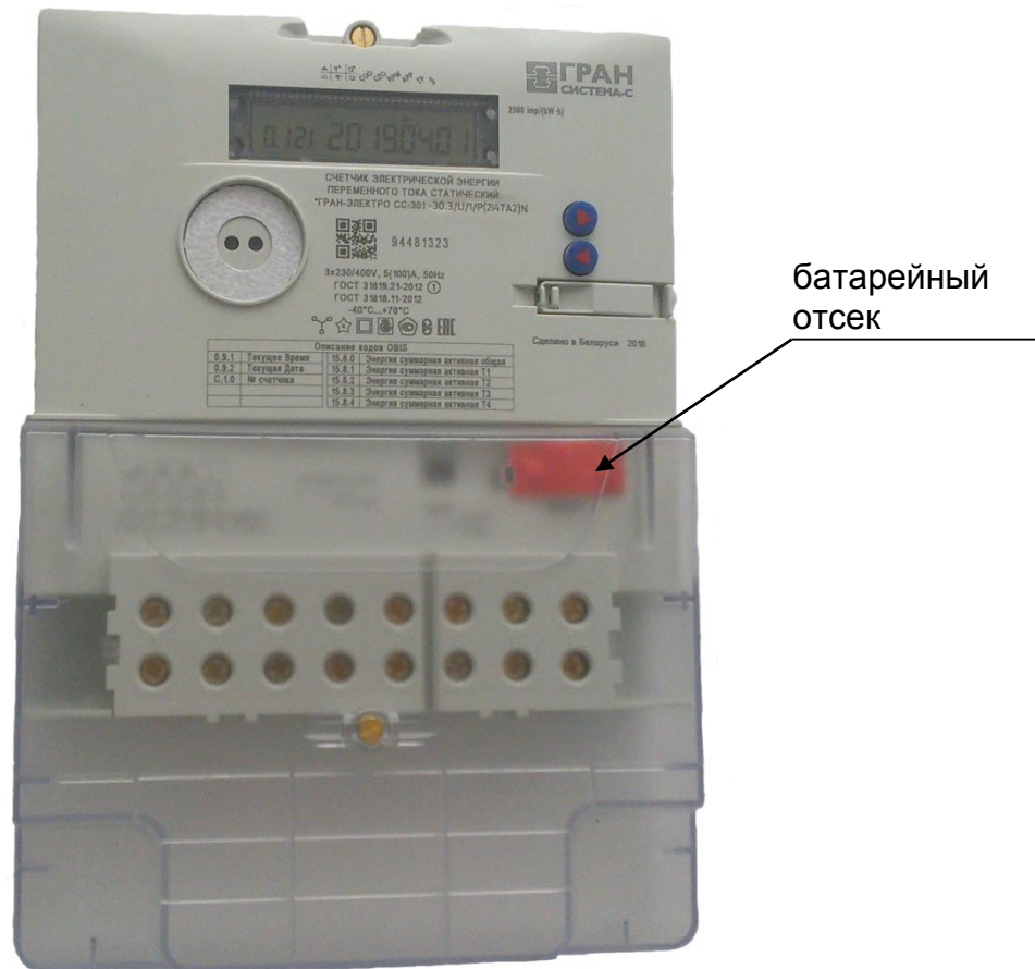
Рисунок 1.3 – Внешний вид счетчиков модификации «Гран-Электро СС-301-Х.Х/У/1/Р(4ТА2Х)N» с прозрачной крышкой
