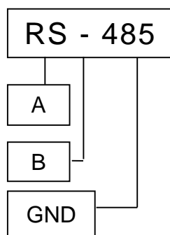
Рисунок Б.2 – Схема подключения счетчика с интерфейсом RS-485
