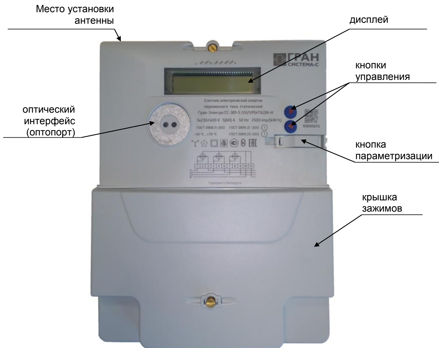
Рисунок 1.2 – Внешний вид счетчиков модификации «Гран-Электро CC-301-Х.Х/U/1/P(4ТА2Х)N»
