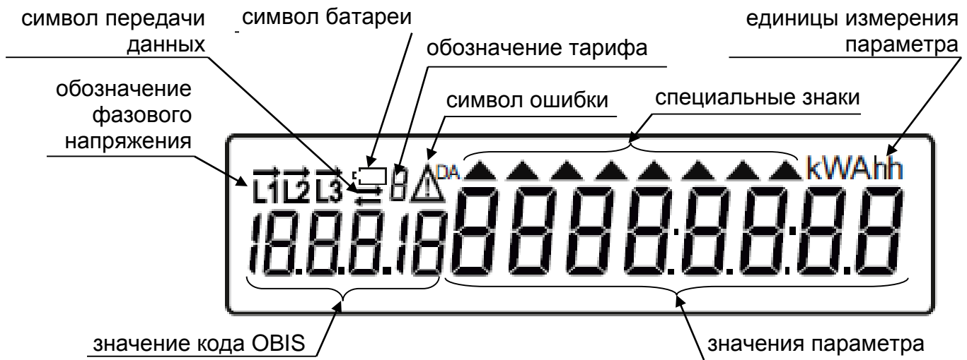
Рисунок 3.1 – Внешний вид дисплея счетчика со всеми включенными сегментами
