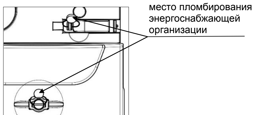
Рисунок В.2 – Место пломбирования энергоснабжающей организации счетчиков (вид с установленной крышкой зажимов)
