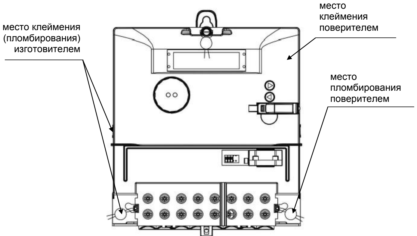
Рисунок В.1 – Защита от несанкционированного вскрытия крышки корпуса (вид корпуса со снятой крышкой зажимов)
